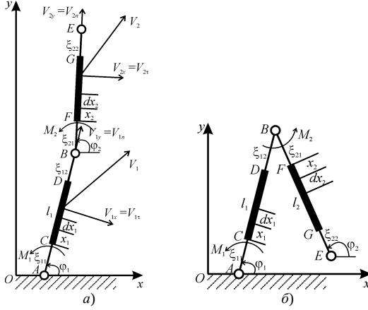
Рисунок 6. Модель двух звеньев экзоскелета переменной длины, шарнирно соединенных между собой
