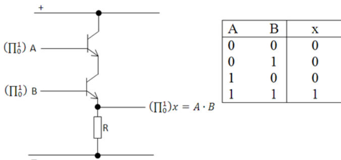
Рисунок 2. Электронная схема для вентиля И
