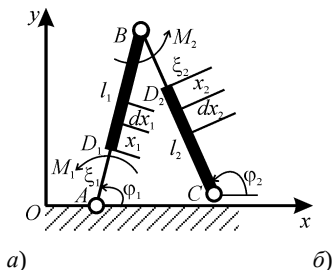
Рисунок 4. Модель двух звеньев экзоскелета переменной длины, шарнирно соединенных между собой
