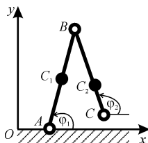
Рисунок 2. Модель экзоскелета с двумя подвижными звеньями
